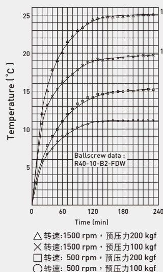
图4.30 工作速度、预压力与温升的关系
