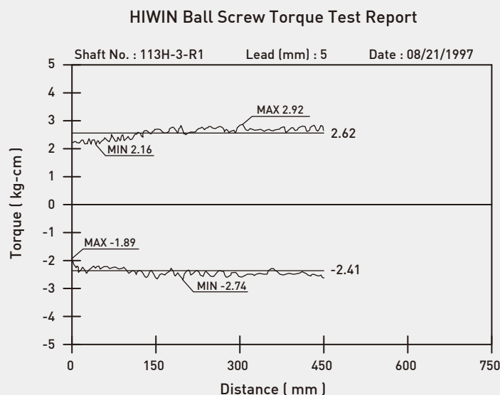
图2.5 HIWIN滚珠丝杠预压扭矩检测图
