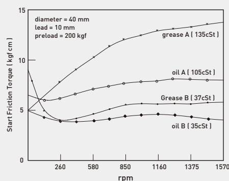
图4.32 摩擦扭矩对油品黏度的影响
