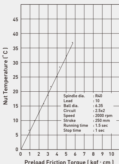
图4.31 温升与预压摩擦扭矩的关系
