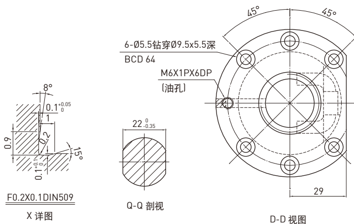
D-D 视图
